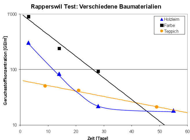
Abb. 1: Zeitlicher Verlauf der Geruchsemissionen von Holzleim, Farbe und Teppich.
